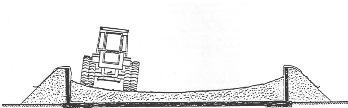
Figuur 11.3 Het hol vullen van een sleufsilos
