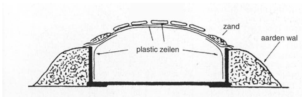
Figuur 11.4 Wijze van afdekken van een sleufsilo met uitsluitend plastic
